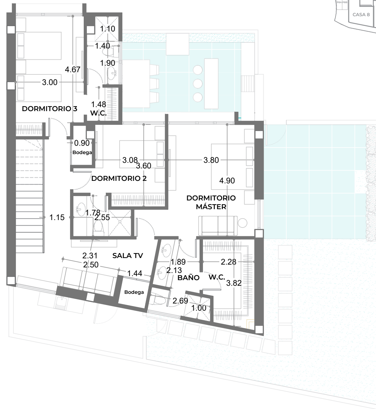
PLANTA ALTA Área: 118.40 m 2
