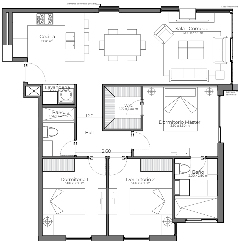
DEPARTAMENTO 204 Construcción: 97.44 m 2
