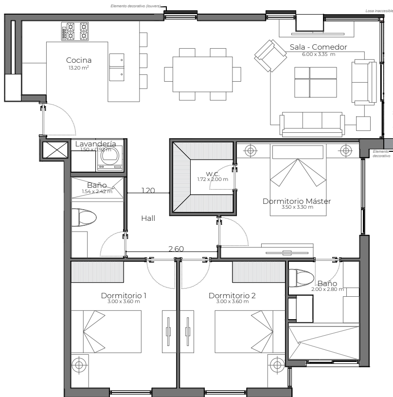
DEPARTAMENTO 304 Construcción: 97.44 m 2
