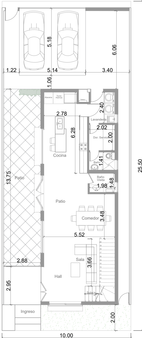
PLANTA BAJA 100.20 m 2
