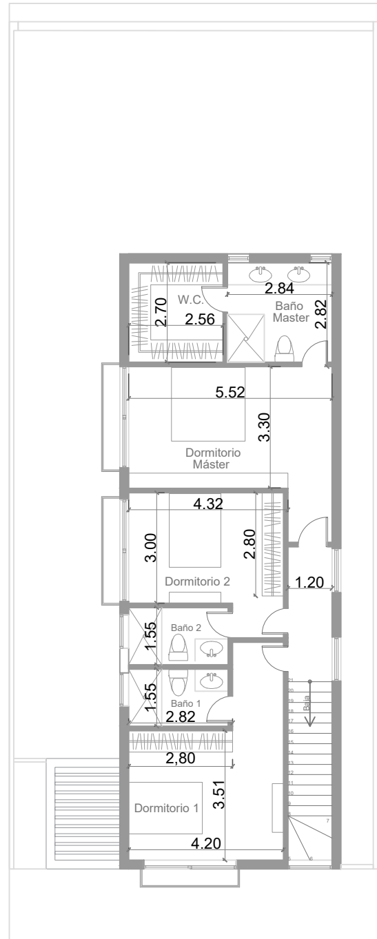
PLANTA ALTA 104.20 m 2
